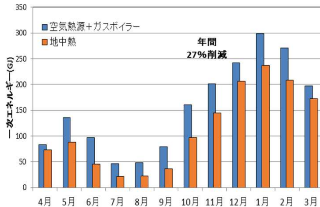
[一次エネルギー消費量] ※2011年4月~2012年3月
