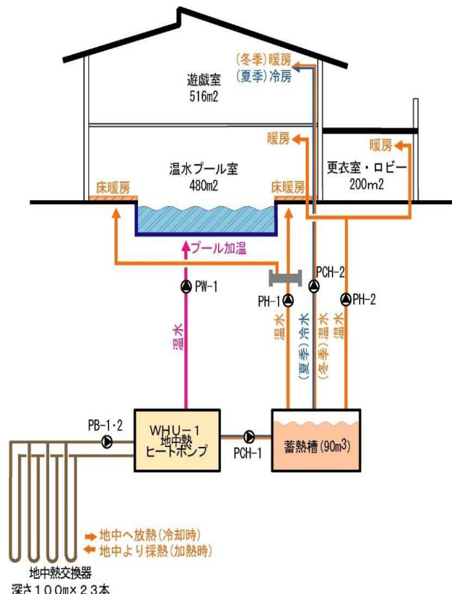
[システム概念図]
