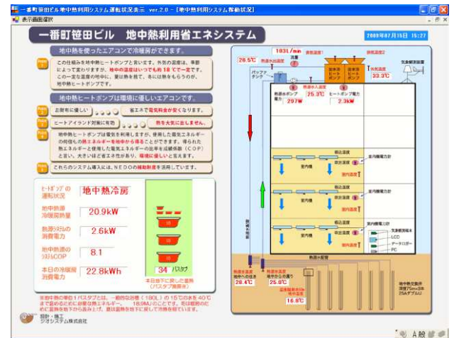
地中熱ヒートポンプの運転状況を常時モニター。データは1分間隔で取得。システムCOP、熱源水温度、利用熱量、地下温度等を表示。
