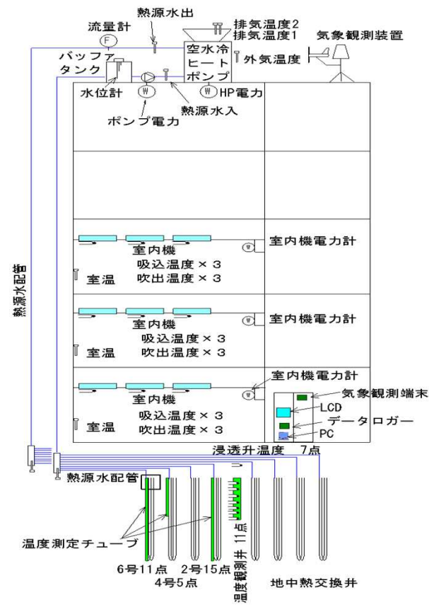
[システム概念図]
