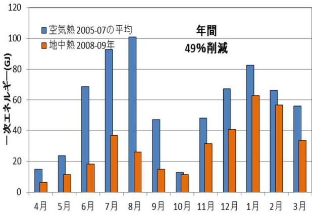
[一次エネルギー消費量] ※2008年4月~2009年3月
